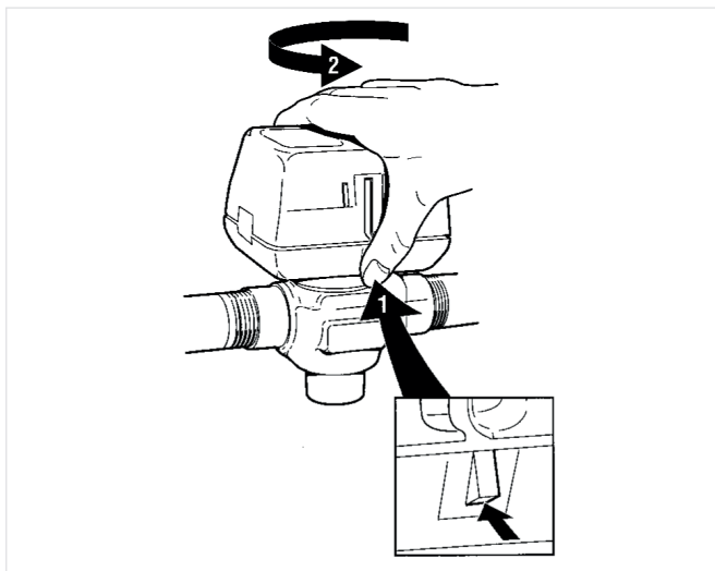
Obr. 6. Západkový mechanismus
